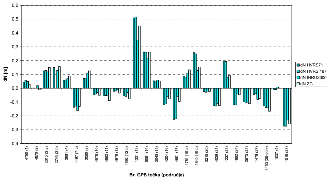
Slika 4. Usporedba reduciranih vrijednosti undulacija dN GPS-točaka ( dN = N_{\text{sred}} - N )
