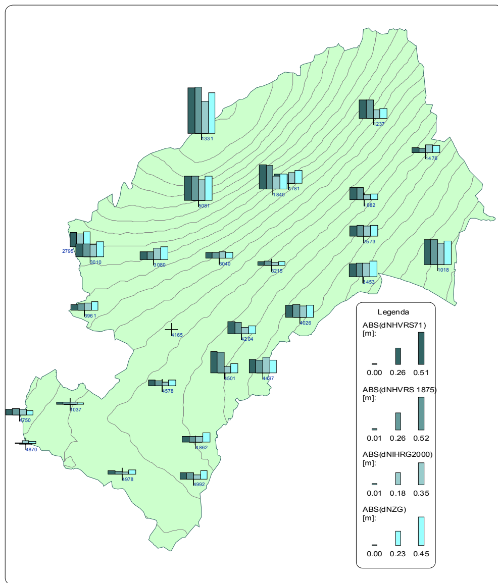
Slika 5. Usporedba reduciranih apsolutnih vrijednosti undulacija, ( dN_{HVRS71} , dN_{HVRS 1875} , dN_{IHRG2000} , dN_{ZG} )
