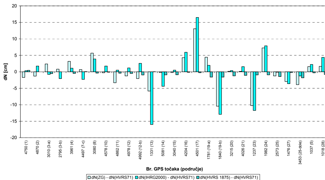
Slika 6. Usporedba razlika reduciranih vrijednosti undulacija ( dN_{ZG}-dN_{HVRS71} , dN_{HRG2000}-dN_{HVRS71} , dN_{HVRS 1875}-dN_{HVRS71} )
