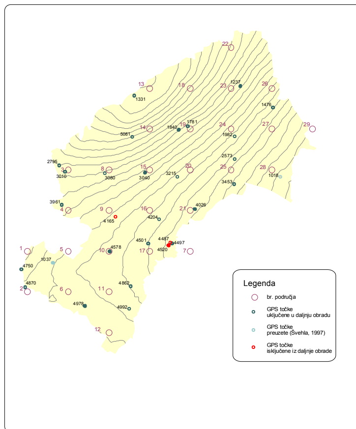
Slika 3. Grafički prikaz područja s GPS/nivelmanskim točkama
