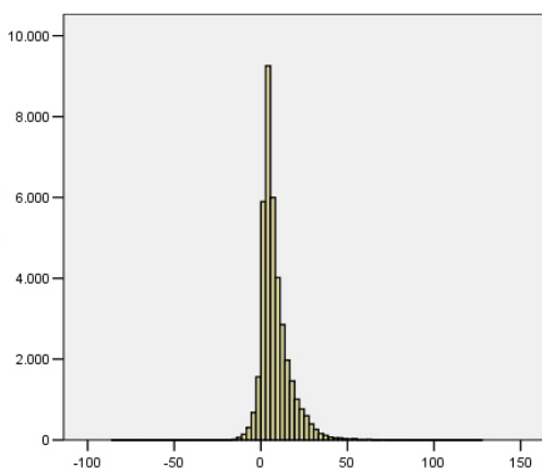
Slika 11. Histogram razlika TRIG-SRTM3x3
