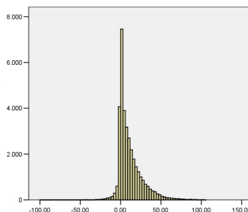
Slika 12. Histogram razlika TRIG-DMR4x5
