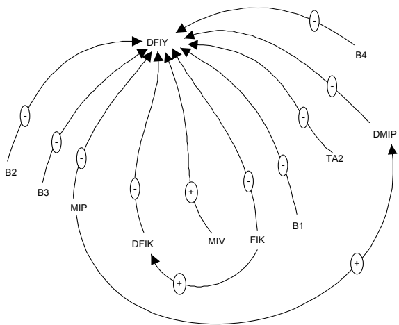
Sl. 3. Strukturni model brodskoga parnog kotla – po razini vode
