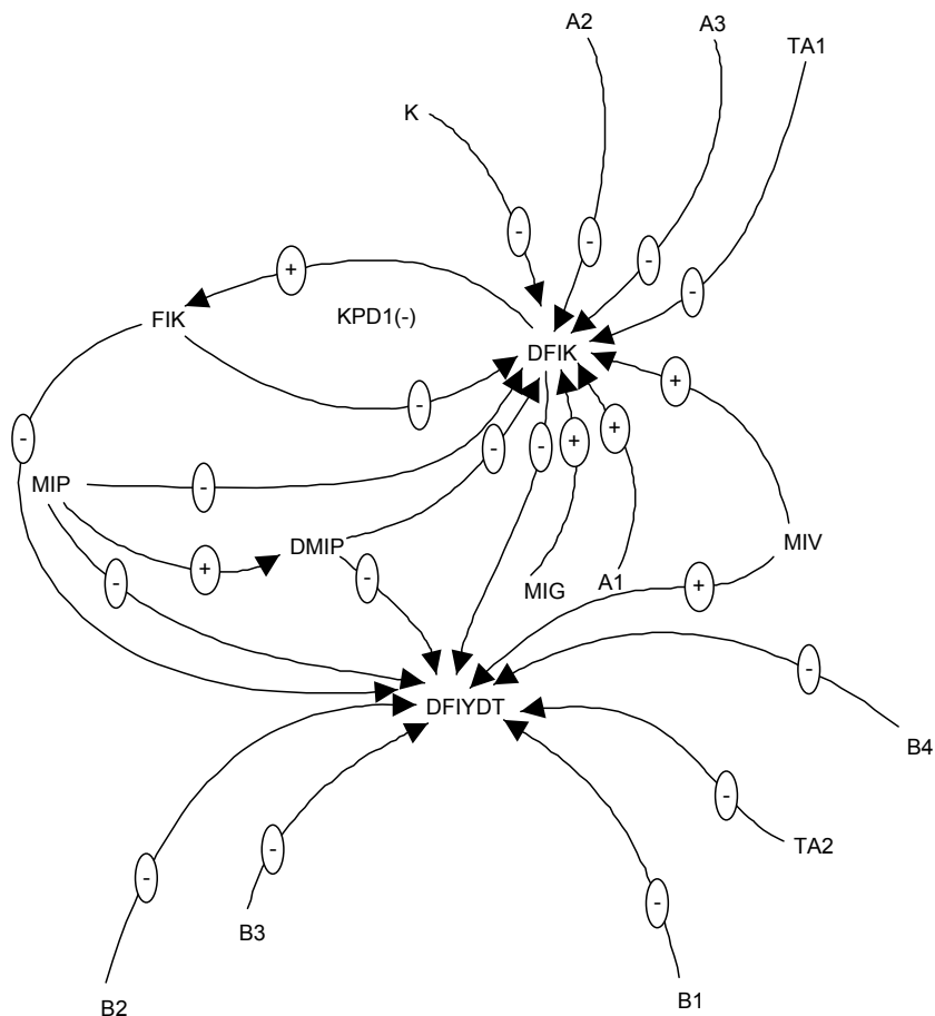
Sl. 4. Globalni strukturni model brodskoga parnog kotla
