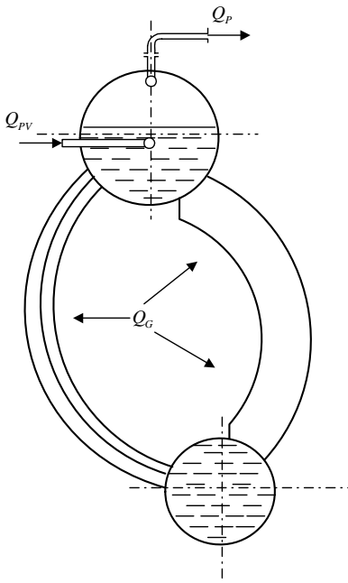
Sl. 1. Prikaz parnog kotla s prirodnom cirkulacijom
