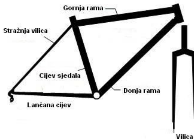
Slika 13. Dijelovi okvira
