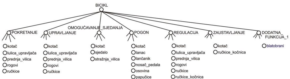
Slika 66. Varijanta bicikla sa blatobranima
