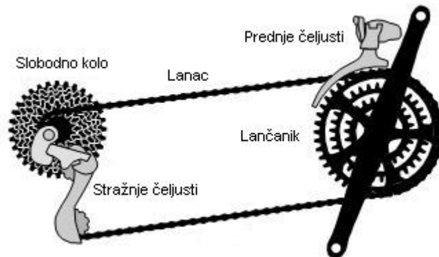
Slika 15. Dijelovi pogona
