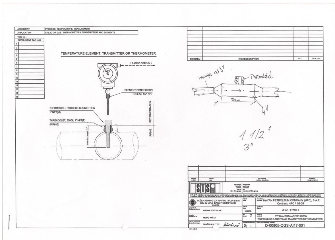
Slika 2.7 Detalj spajanja termometra [8]
