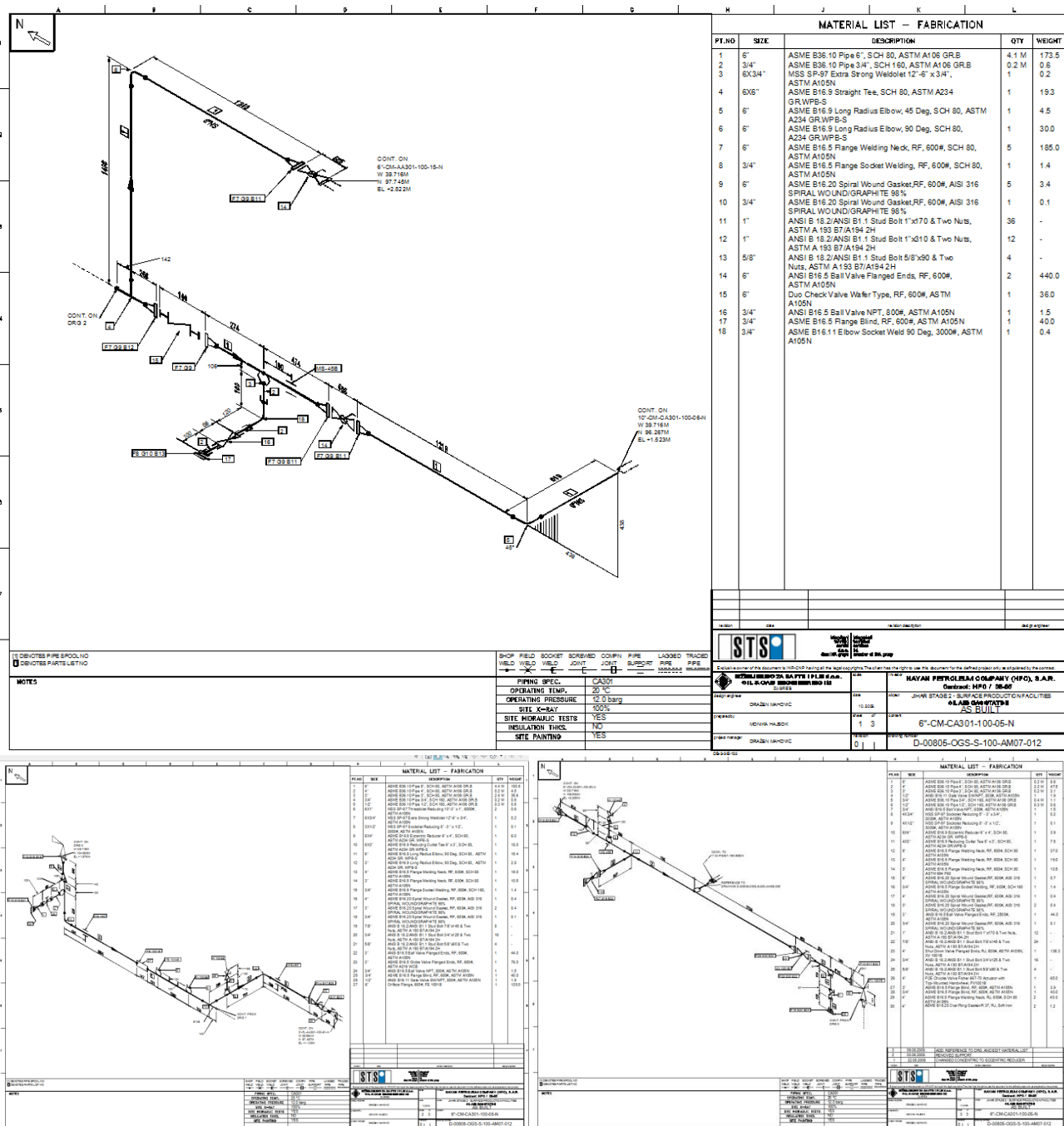
Slika 4.5 Generirane izometrije cijevne linije u DWG formatu [7]
