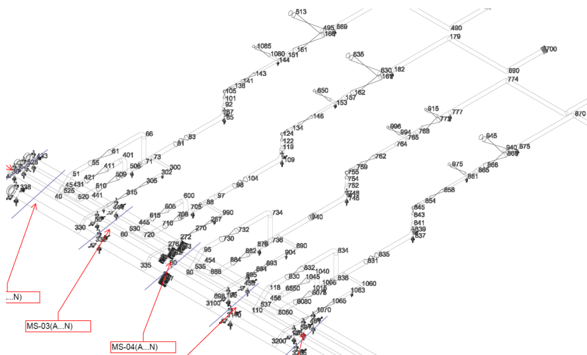
Slika 4.2 Prikaz rezultata analize naprezanja [8]
