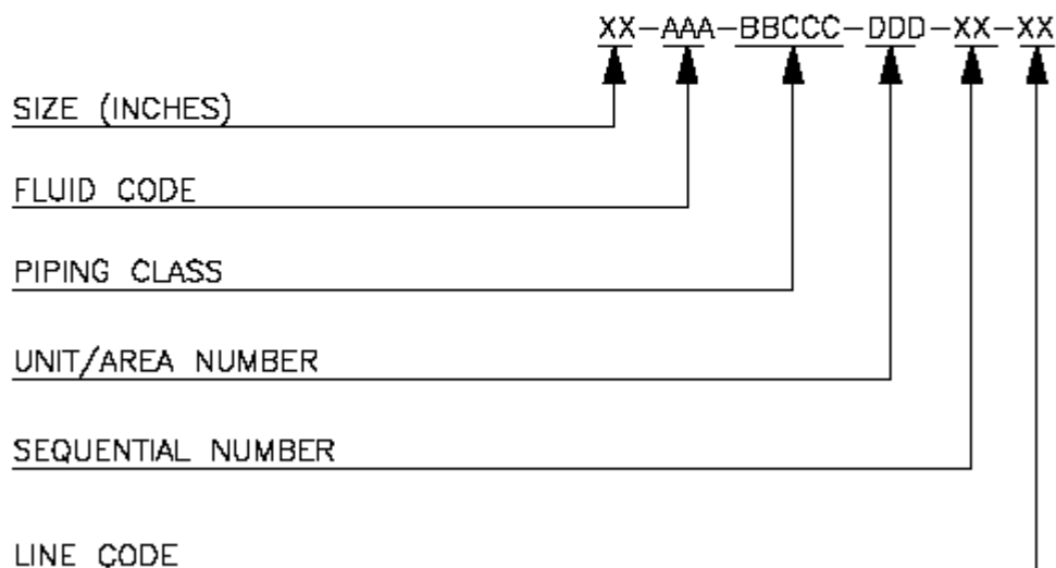
Slika 2.2 Označavanje cijevne linije [5]
