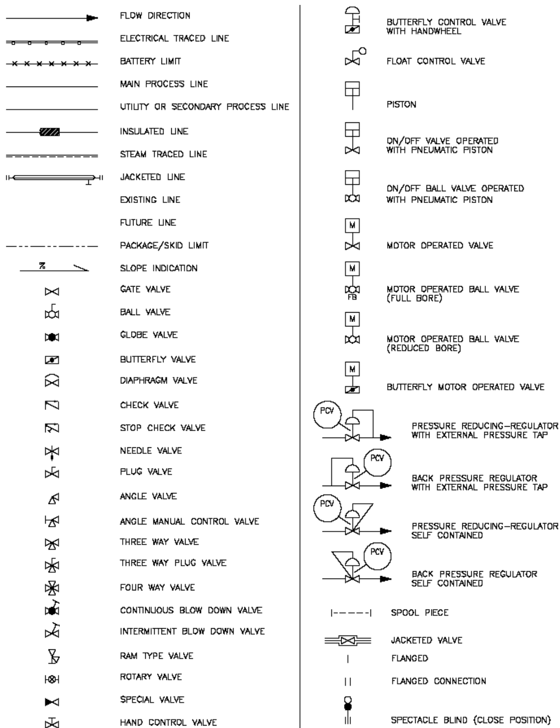
Slika 2.3 Izvorni tumač simbola [5]
