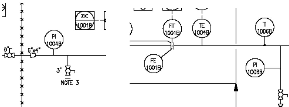
Slika 2.5 Primjer označavanja mjerača za tlak i temperaturu [5]
