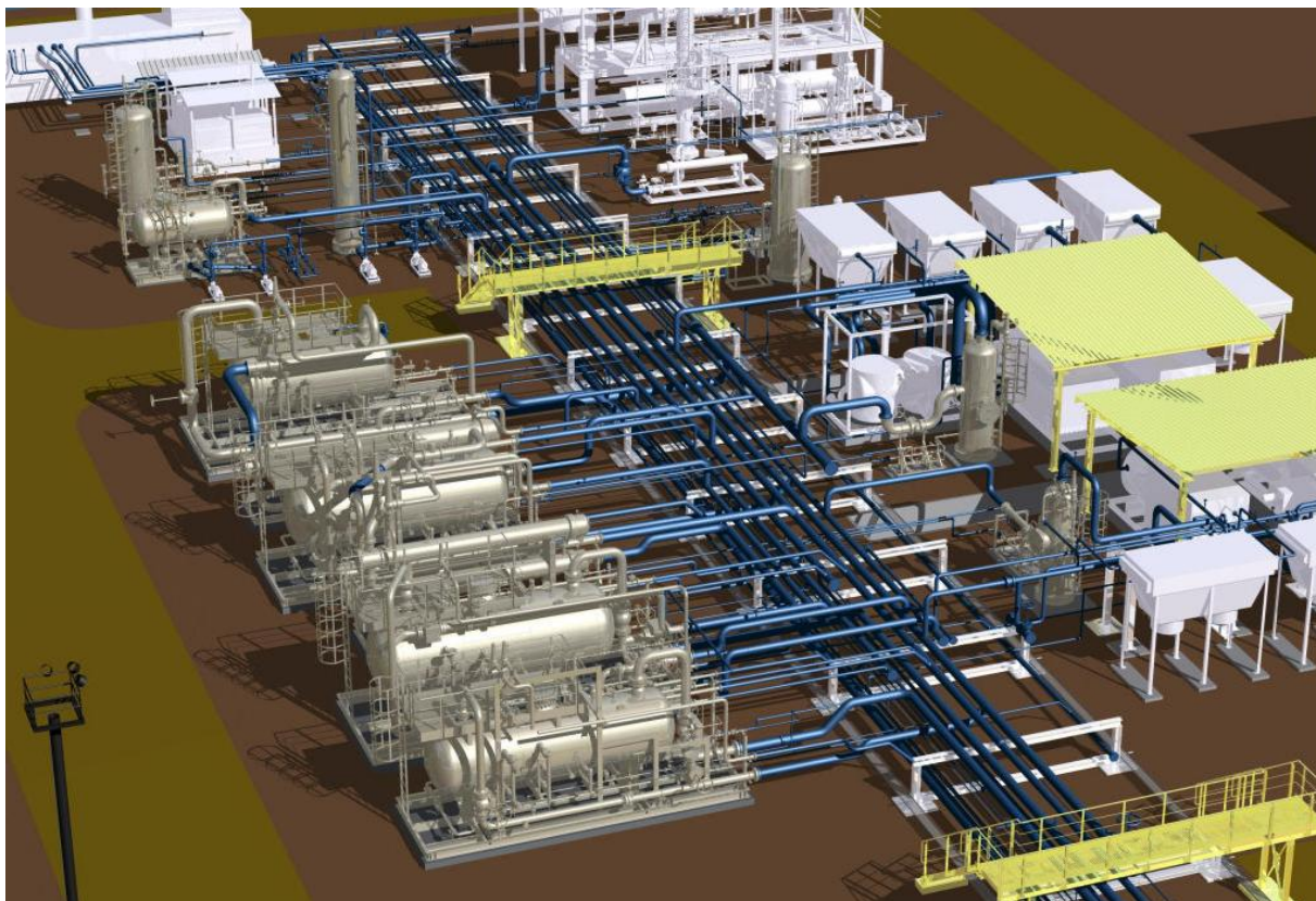
Slika 5.1 Model postrojenja Jihar Faza 2 u Siriji
