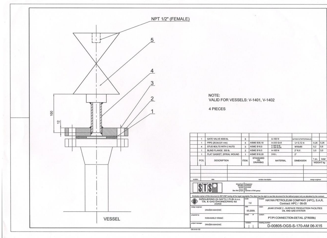
Slika 2.6 Detalj spajanja manometra [8]
