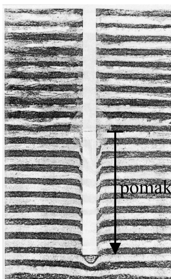
Slika 5.33b Pilot promjera 2,54 cm zabijen s dubine od 25cm na dubinu od 48,3cm u jako zbijenom pijesku ( D_r \sim 0,9 ). Vidljive su deformacije nastale posmičnim napreznjima po plaštu kao i aktivni klin ispod vrha.
