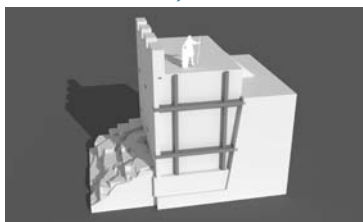
3. Zapadni bedem, vizualizaciju načinio D. Popović prema rekonstrukciji K. Rončevića
