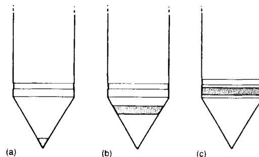
Slika 3.20 Položaj filtra za mjerenje pronažnog pritiska: a) u vrhu, b) u pola visine šiljka, c) neposredno iznad šiljka
