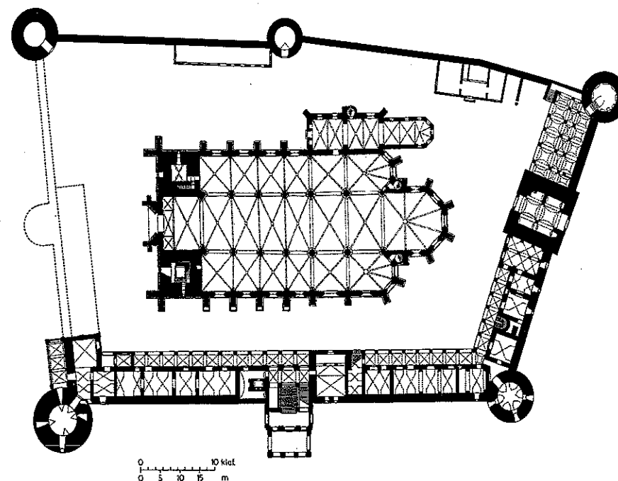
Katedrala i njezina utvrda, tlocrt prizemlja (arh. snimak, I. Tenšek, 1995).
