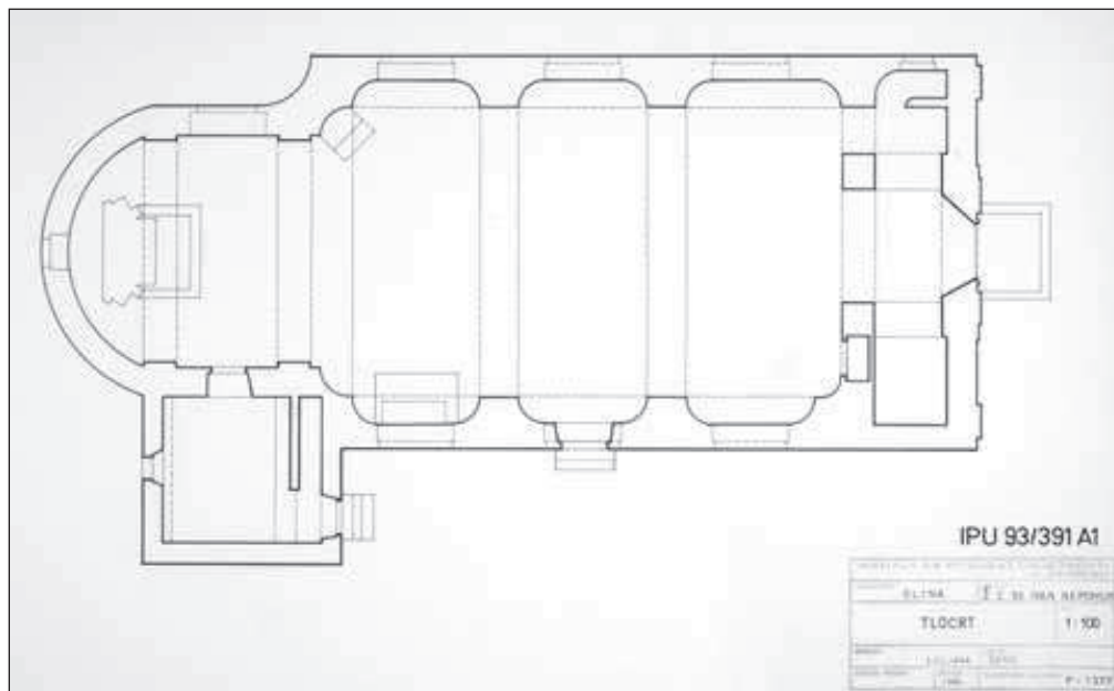
Ilustracija 2. Tlocrt crkve sv. Ivana Nepomuka.
