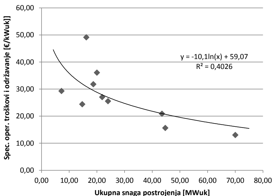
Slika 23. Ovisnost specifičnih operativnih troškova i troškova održavanja o veličini postrojenja na biomasi
