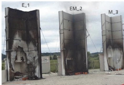
Slika 15. 57 minuta nakon početka – izvor topline je izgorio
