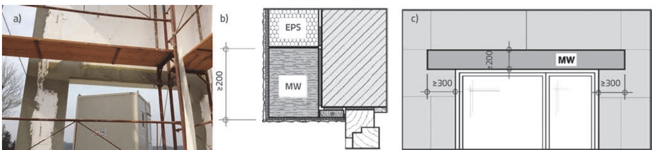
Slika 5. Protupožarna barijera: a) postavljena na uzorku EM_2; b) shema - presjek [14]; c) shema - pogled [14]
