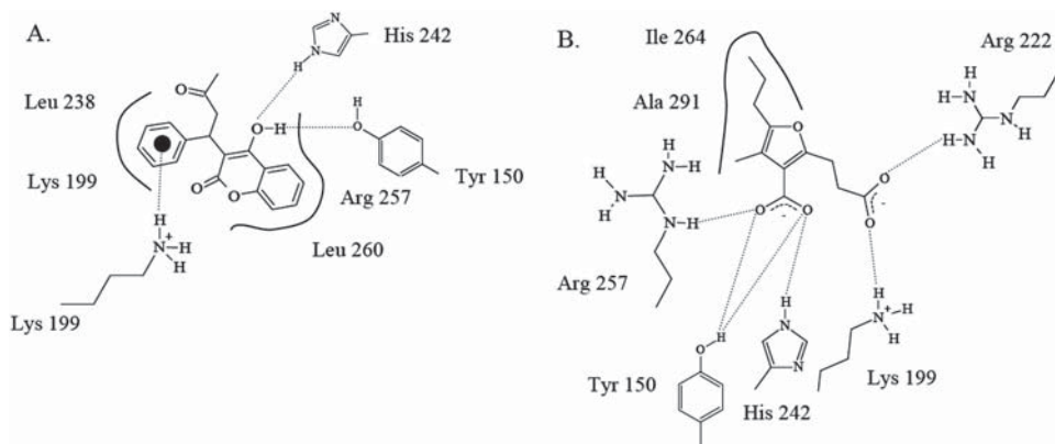
Slika 3. Interakcije između A. varfarina (PDB unos 2BXD) i B. 3-karboksi-4-metil-5-propil-2-furanpropionata (CPMF) s veznim mjestom I (PDB unos 2BXA) (8)
