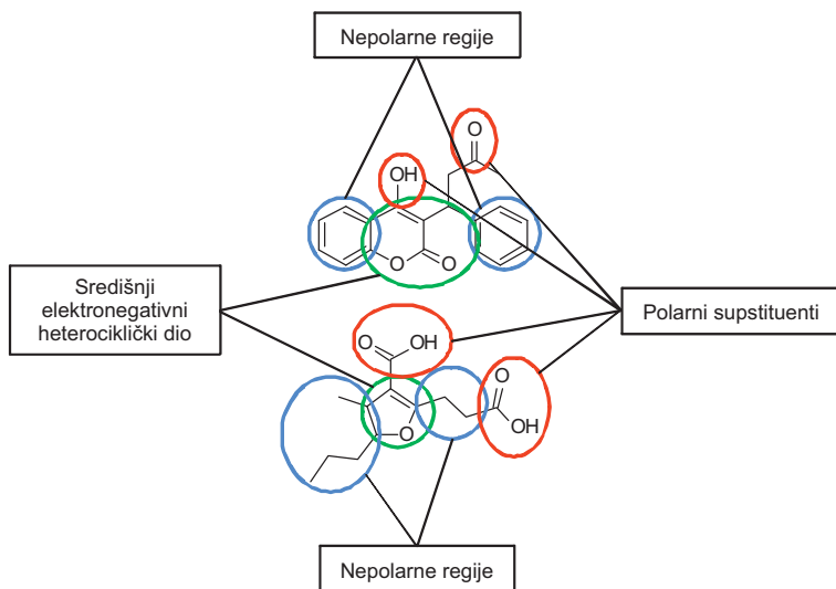
Slika 2. Strukturna svojstva varfarina (gore) i 3-karboksi-4-metil-5-propil-2-furanpropionata (CPMF) (dolje)
