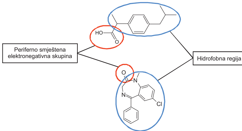
Slika 6. Strukturna svojstva ibuprofena (gore) i diazepama (dolje)
