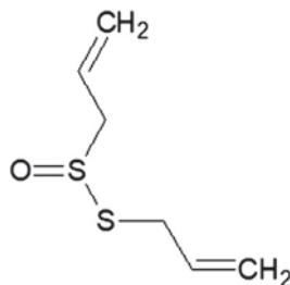
Slika 2. Struktura alicina
