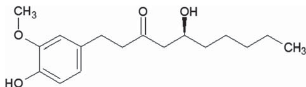
Slika 11. Struktura 6-gingerola
