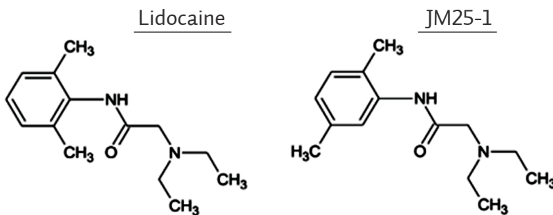
Slika 1. Molekularna struktura lidokaina i JM25-1. Preuzeto i prilagođeno iz [7].
